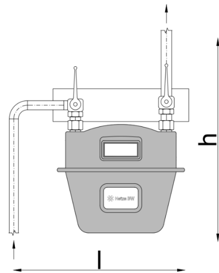
Abbildung 7: Montagebeispiel Balgengaszähler
