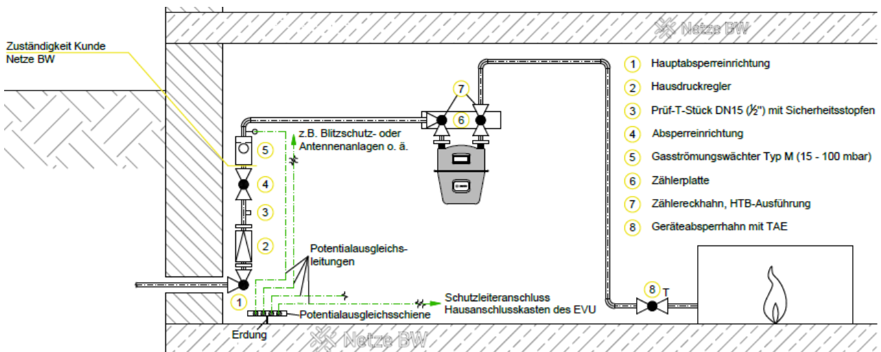
Abbildung 13: Installationsschema Mitteldruck
