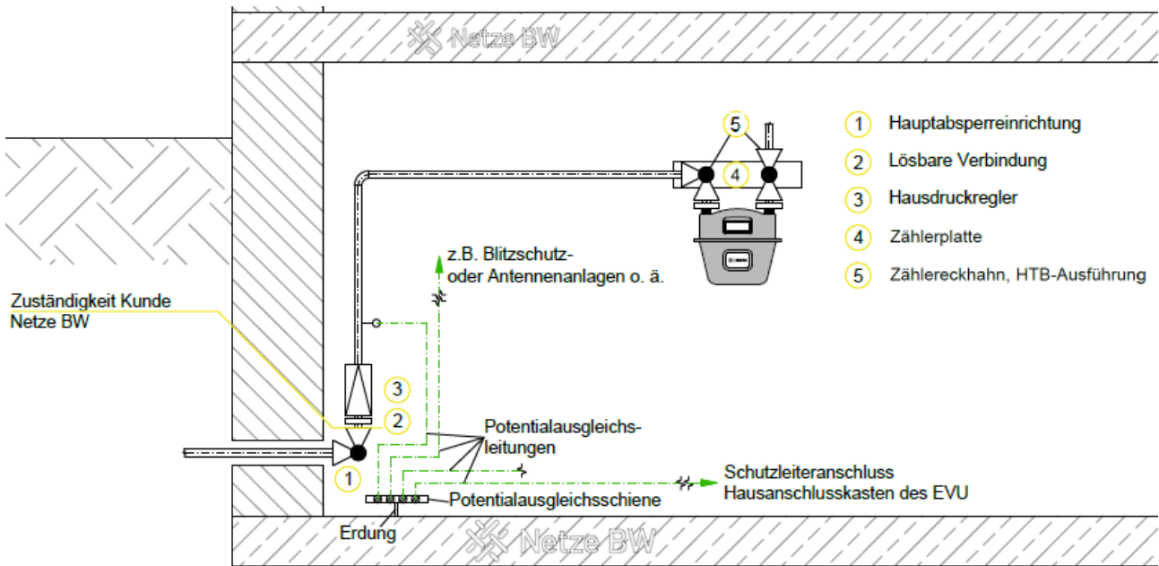
Abbildung 12: Installationsschema Niederdruck mit Hausdruckregelgerät ab Zählergröße G16
